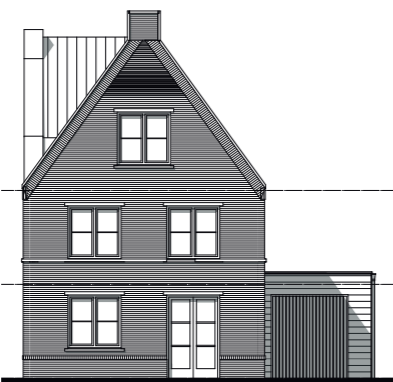
Gevelaanzichten voorgevel
