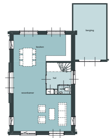
Plattegronden begane grond
