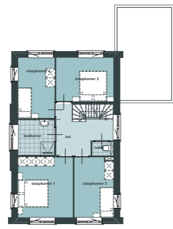
1e verdieping
