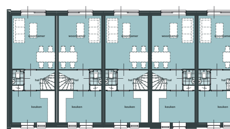
Plattegronden begane grond
