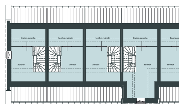
2e verdieping
