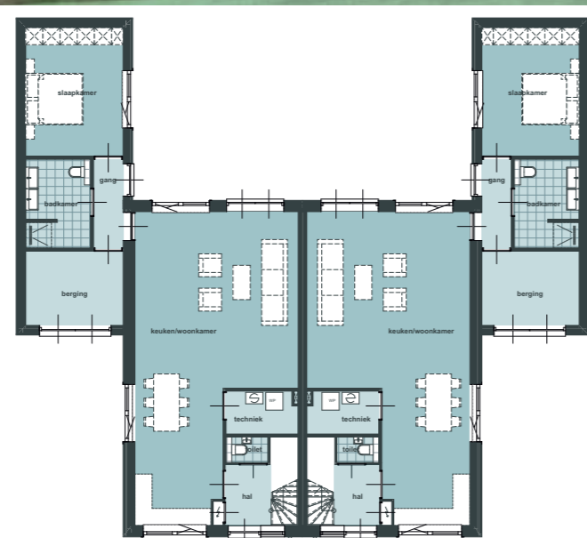
Plattegronden begane grond
