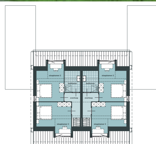
1e verdieping
