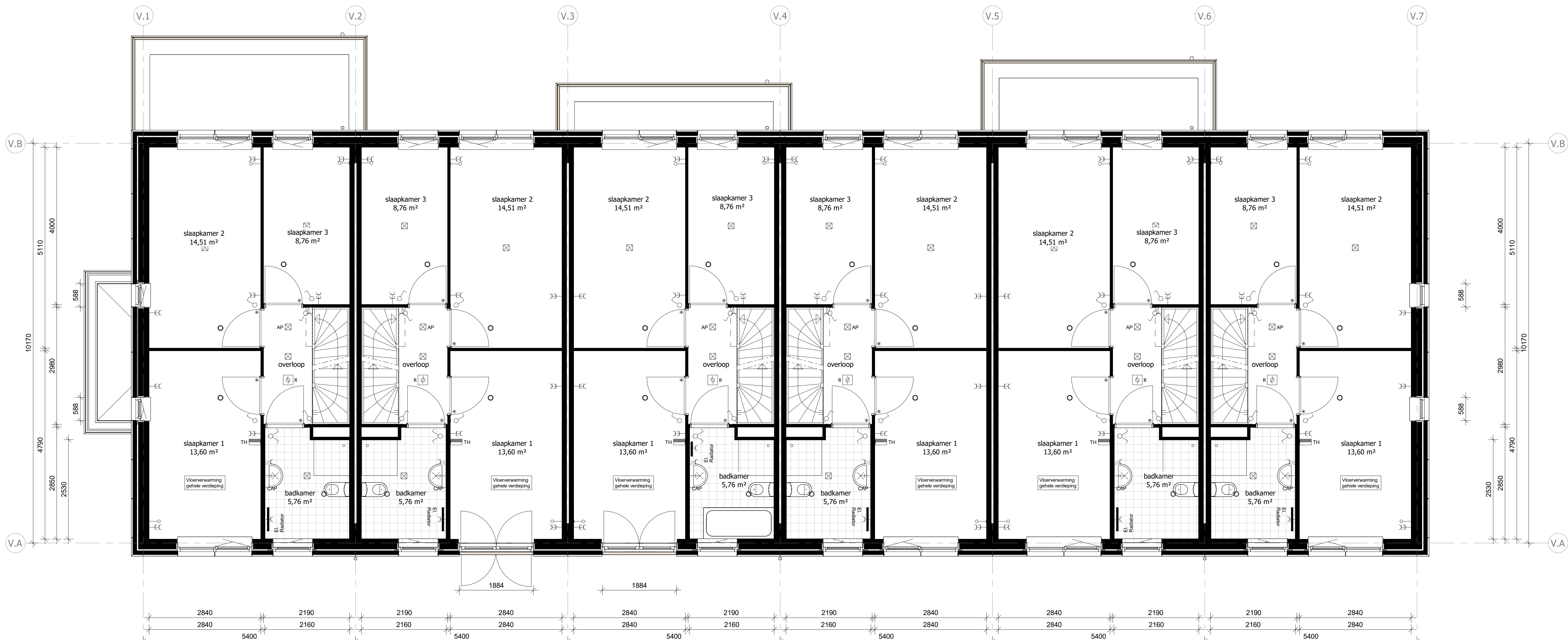
eerste verdieping
