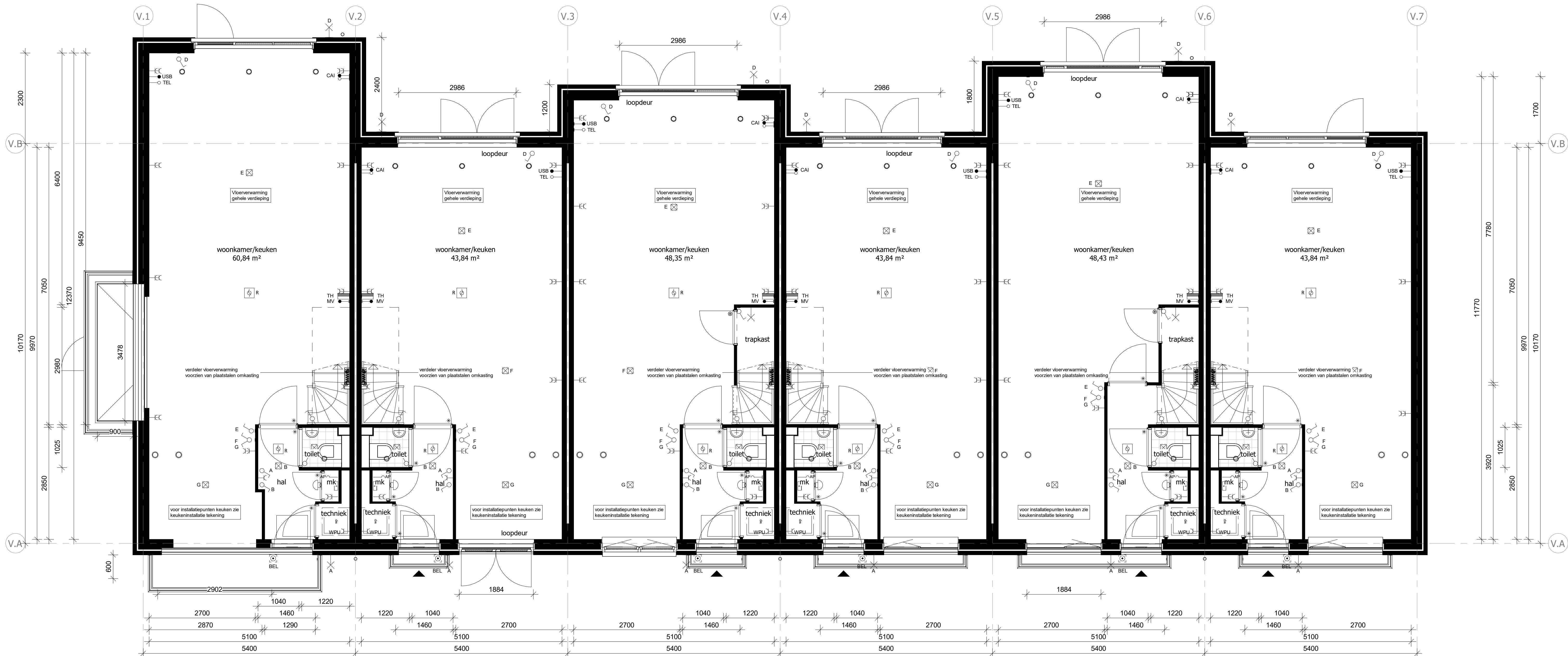
begane grond
