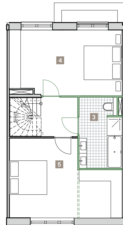
Eerste verdieping
