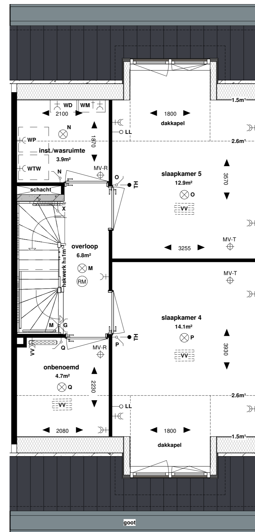
Bnr. 09 - 2e verdieping
