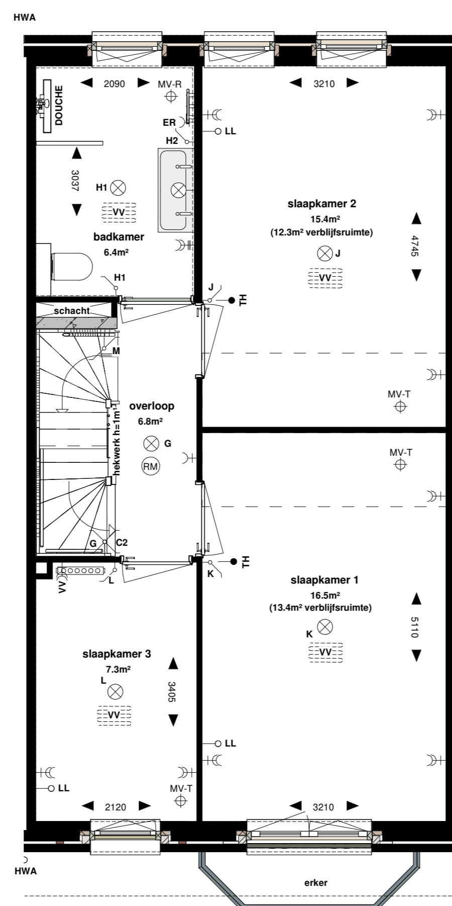
Bnr. 09 - 1e verdieping
