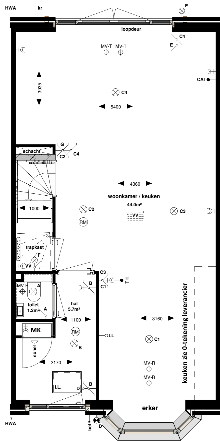
Bnr. 09 - begane grond
