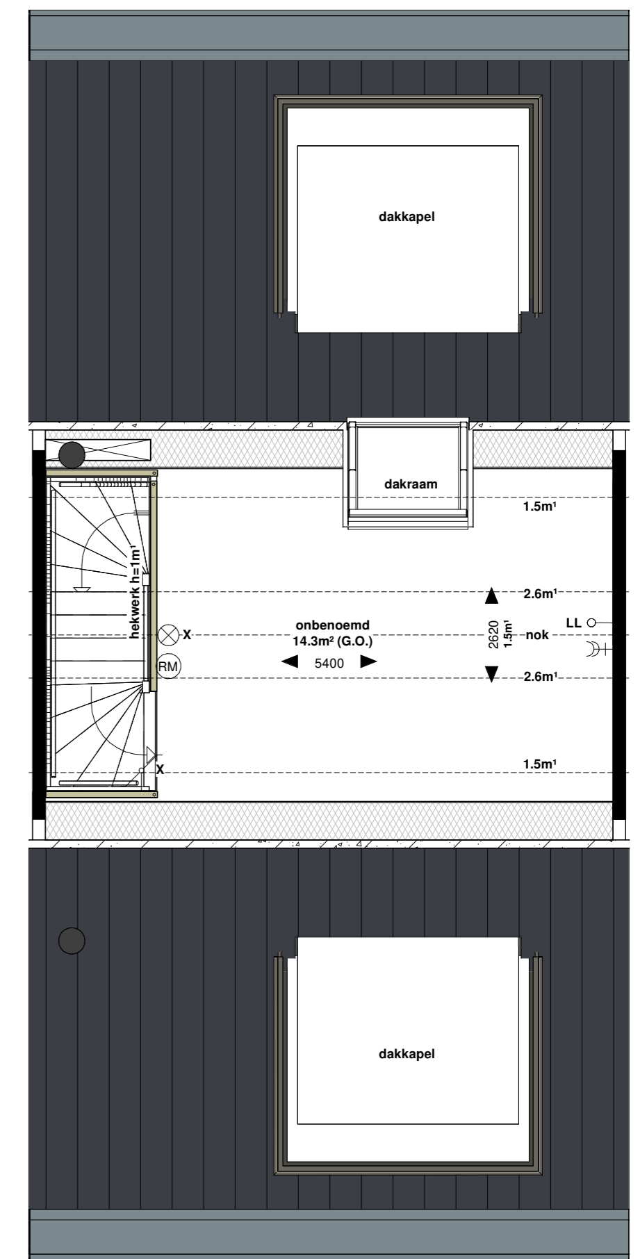
Bnr. 09 - 3e verdieping
