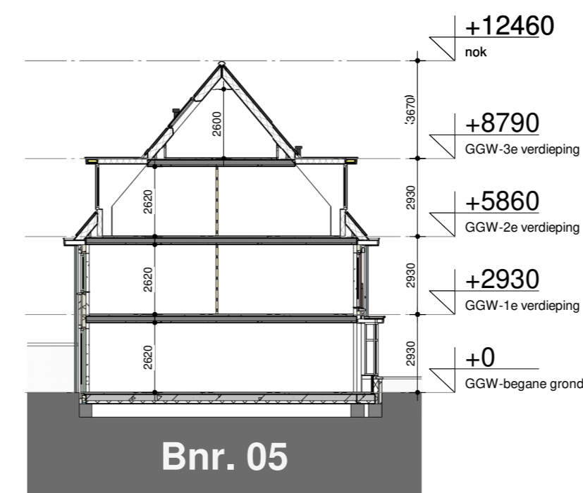
doorsnede
