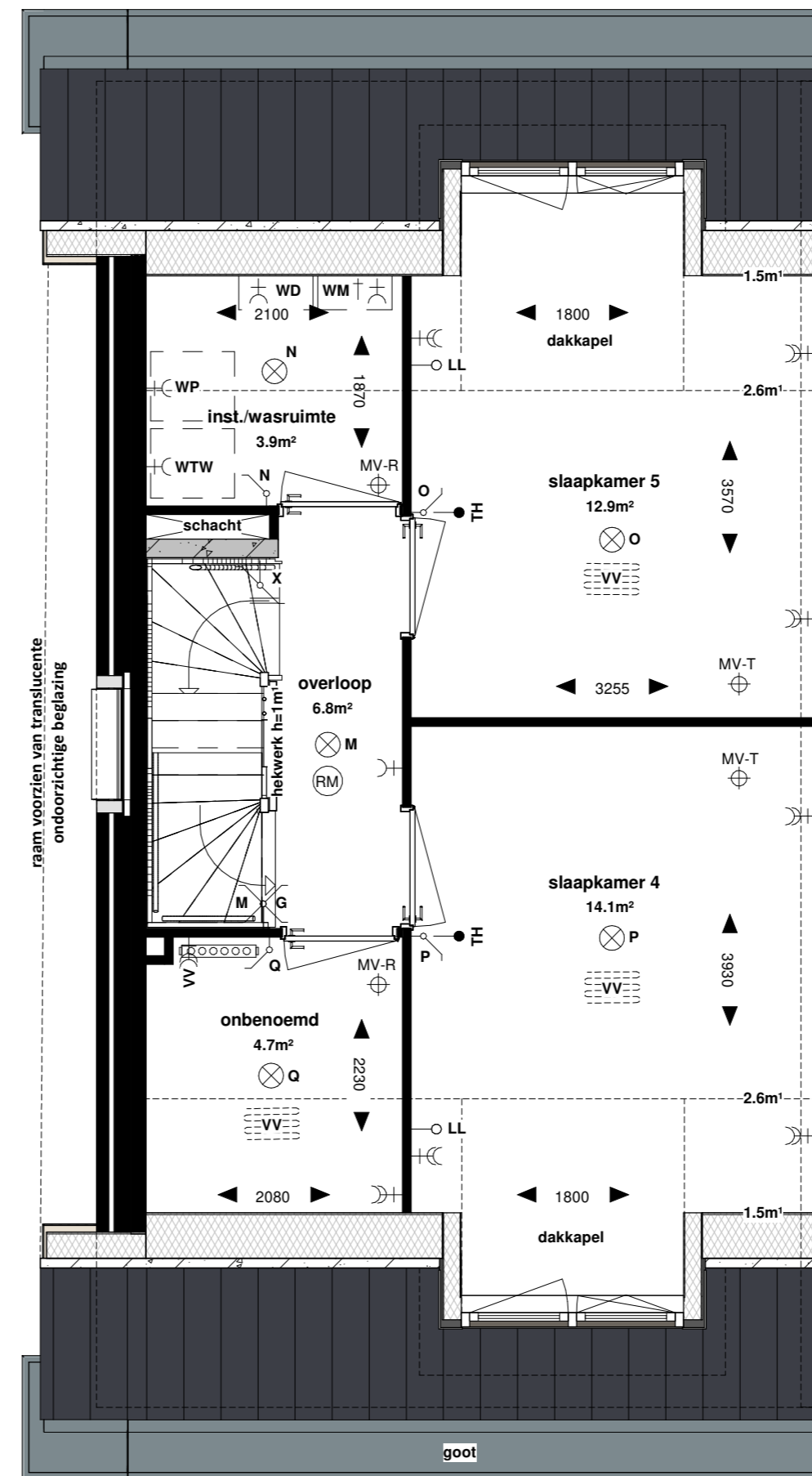
Bnr. 03 - 2e verdieping
