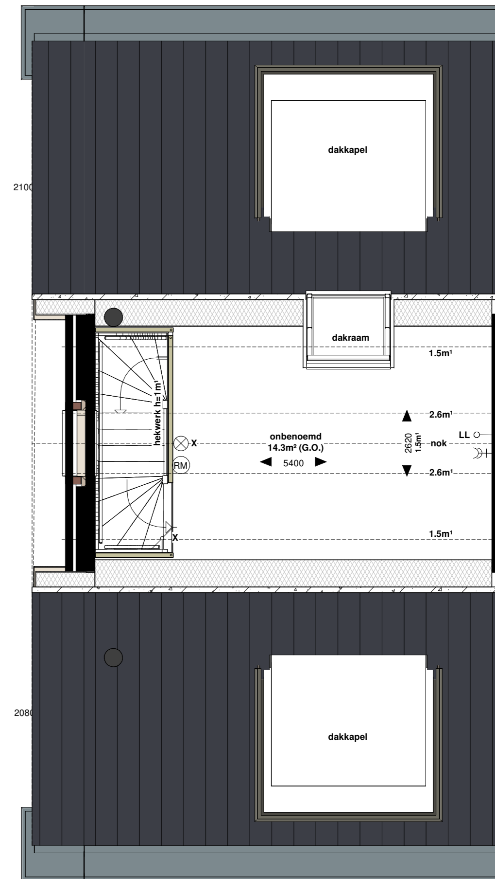
Bnr. 03 - 3e verdieping
