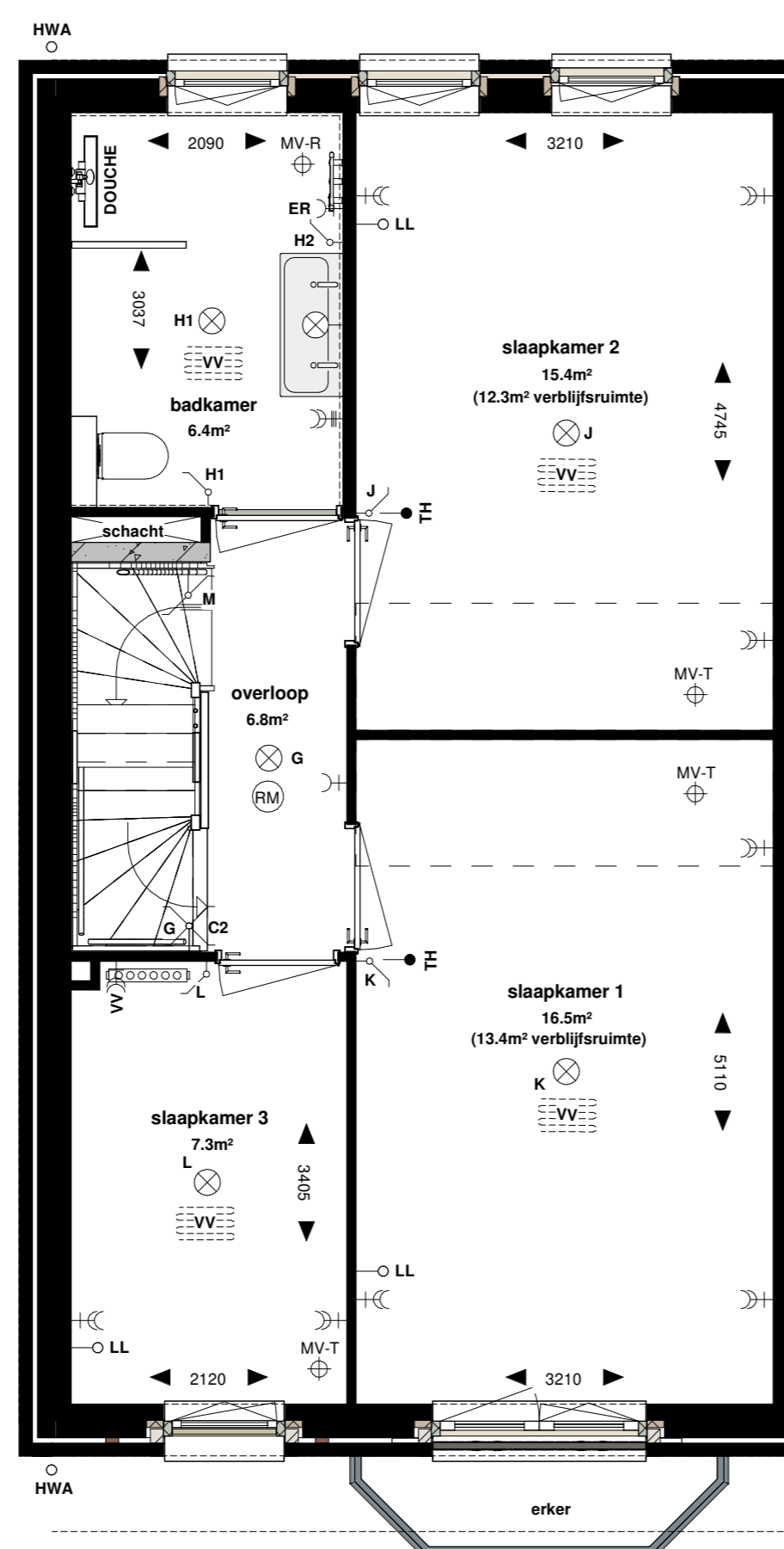
Bnr. 03 - 1e verdieping
