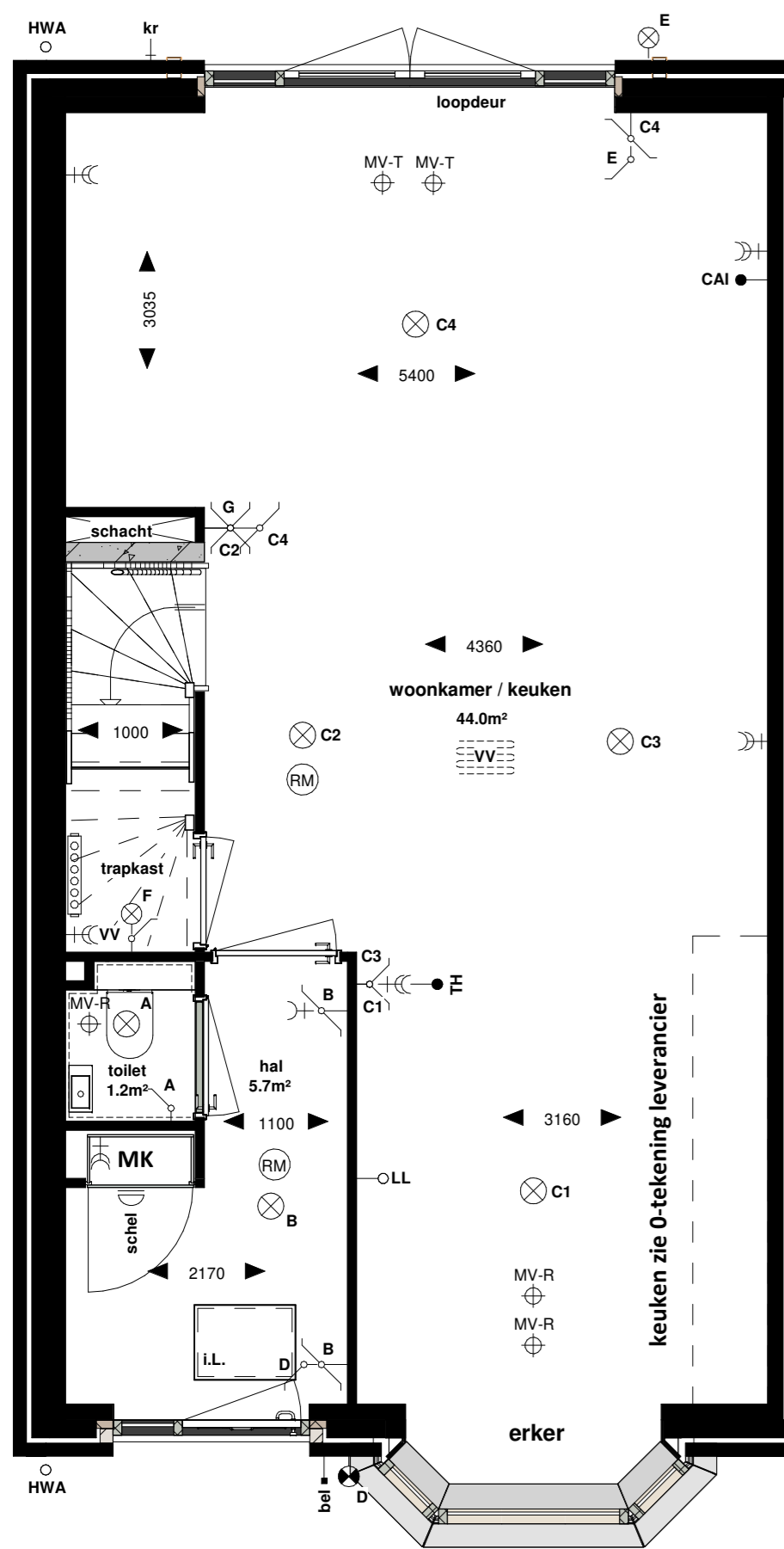
Bnr. 03 - begane grond
