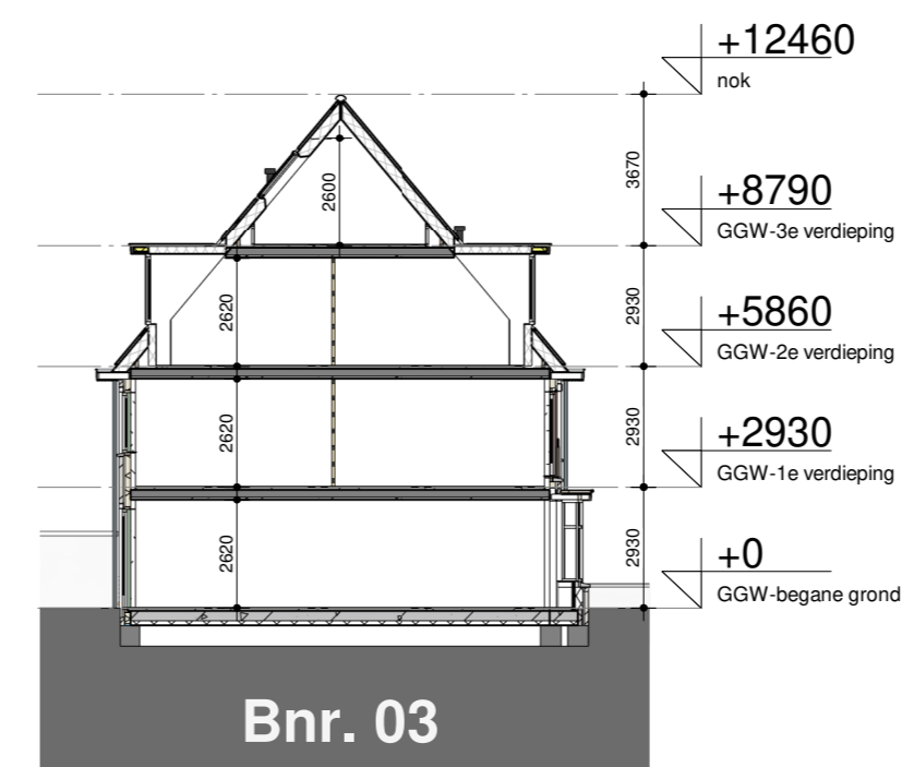
doorsnede
