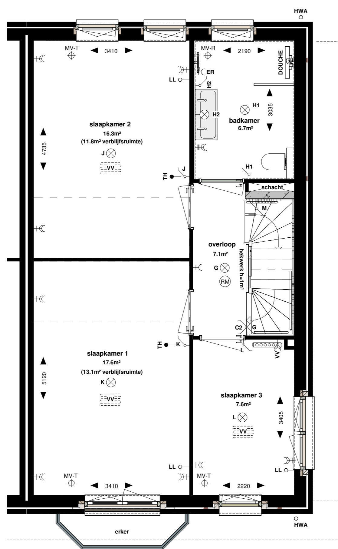
Bnr. 02 - 1e verdieping
