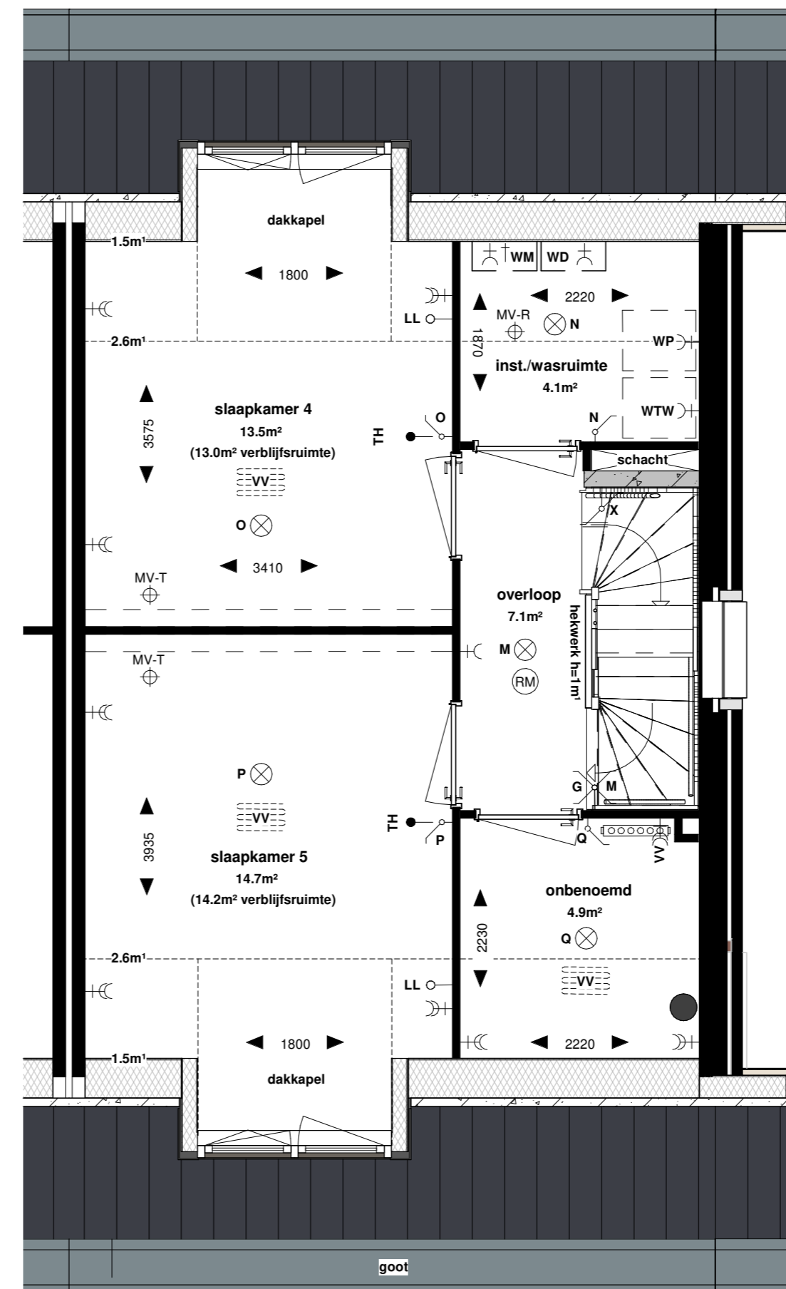
Bnr. 02 - 2e verdieping
