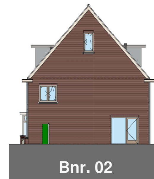
zijgevel rechts
