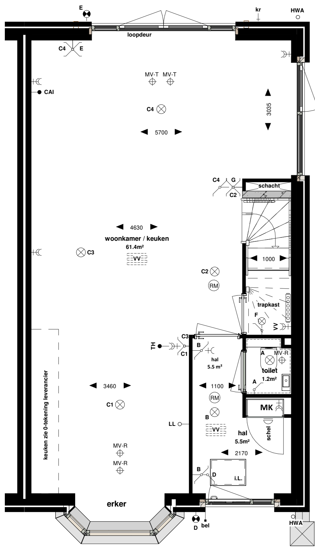
Bnr. 02 - begane grond
