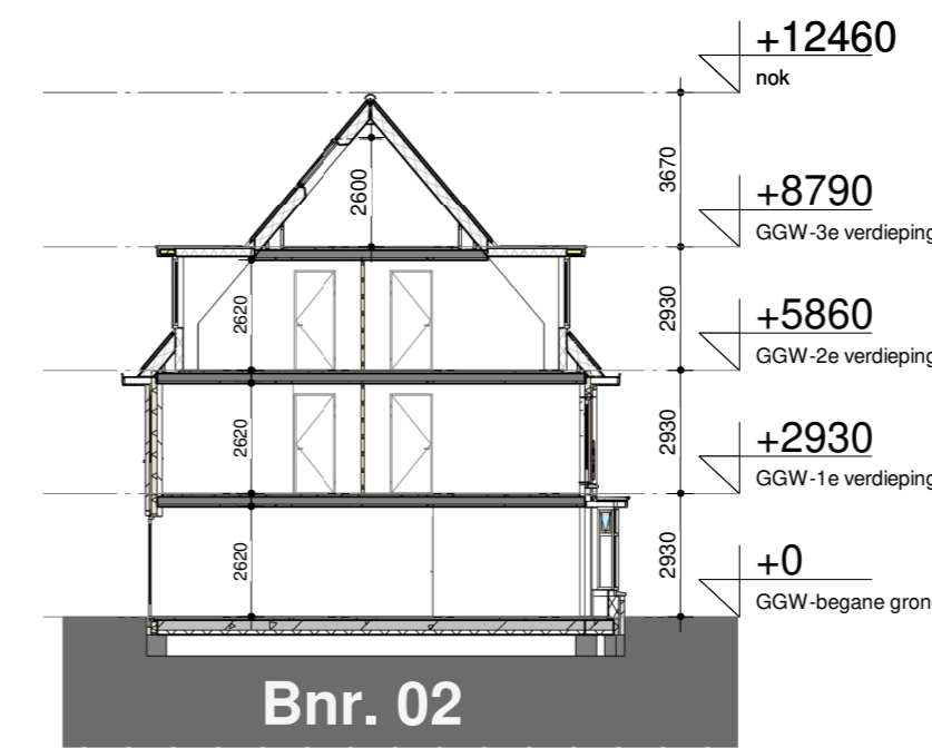
doorsnede
