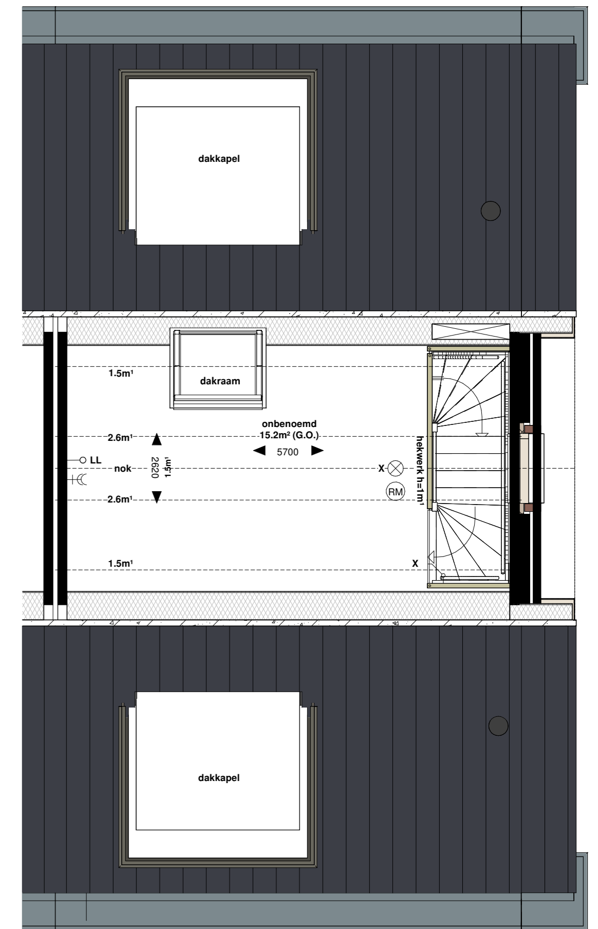
Bnr. 02 - 3e verdieping
