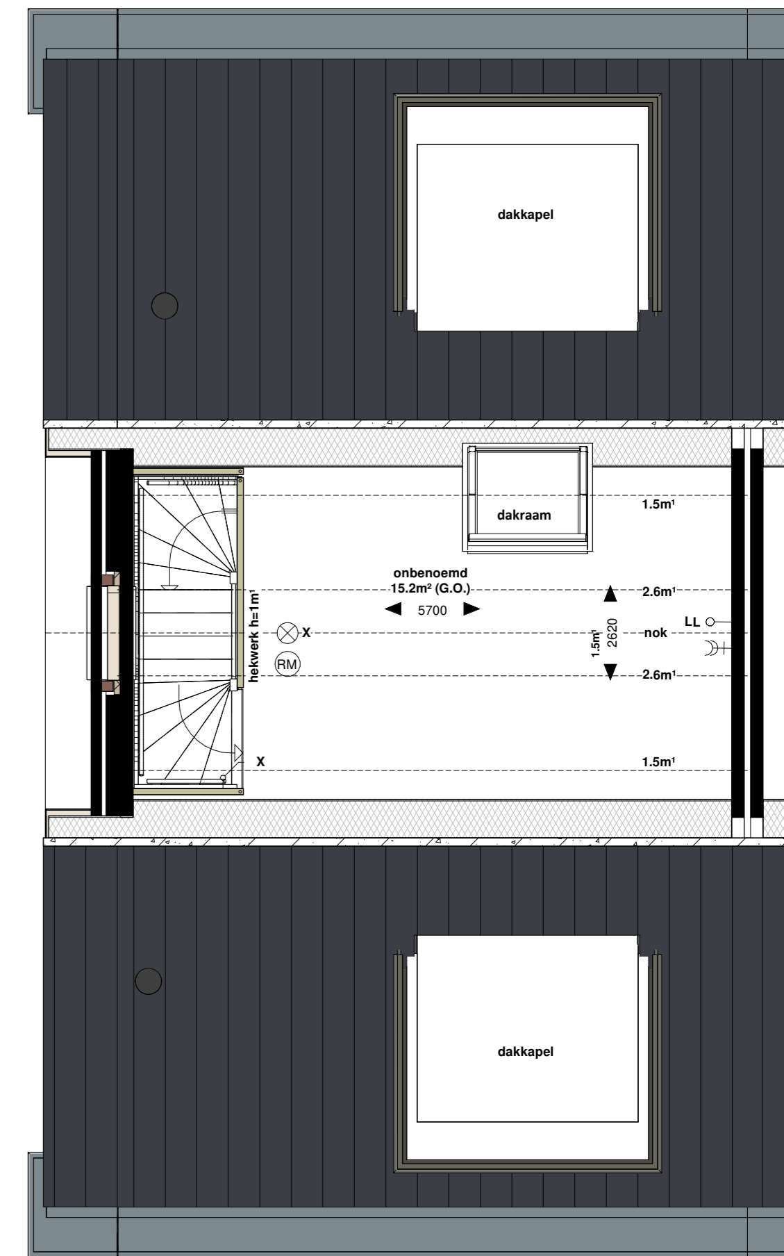
Bnr. 01 - 3e verdieping
