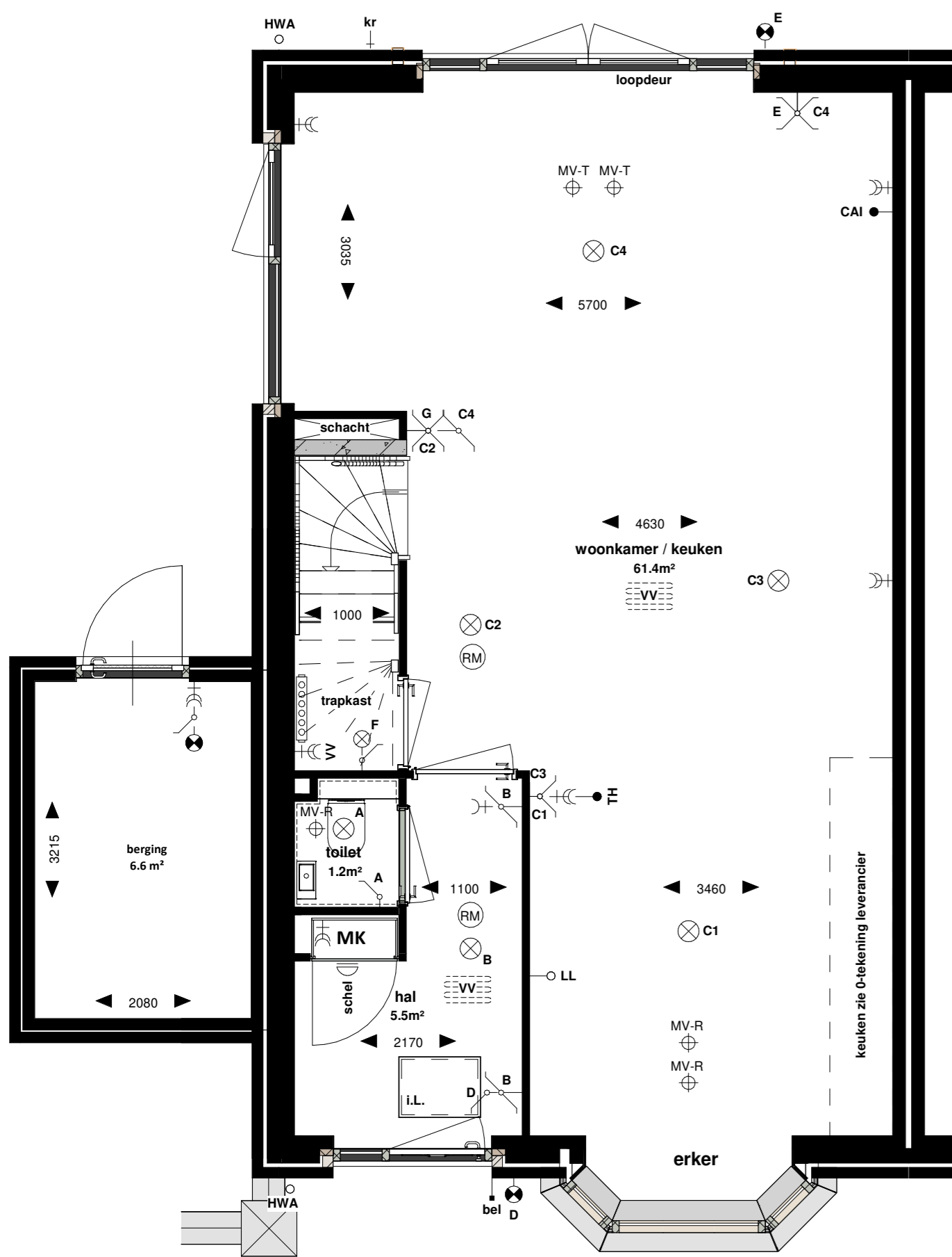
Bnr. 01 - begane grond
