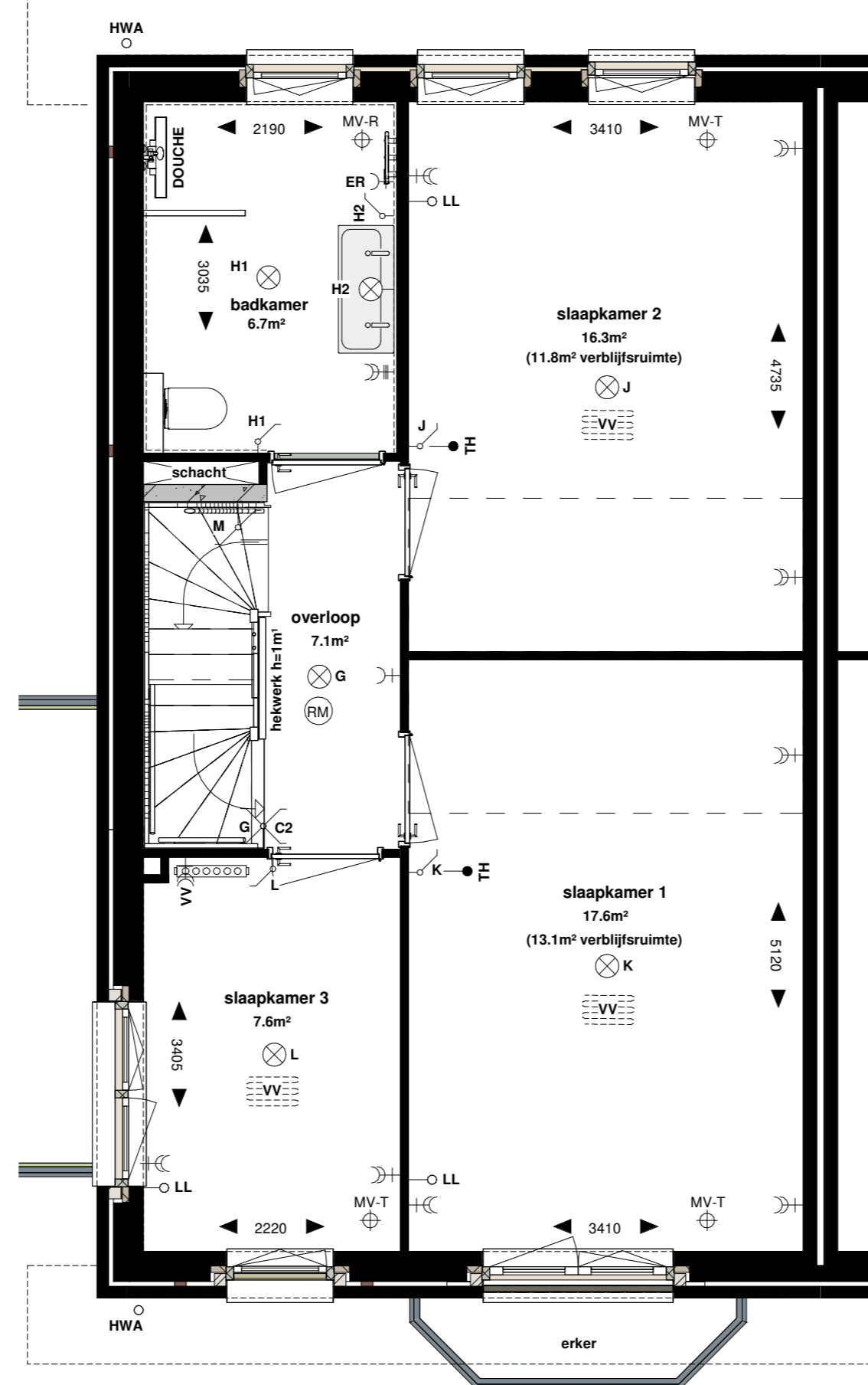
Bnr. 01 - 1e verdieping
