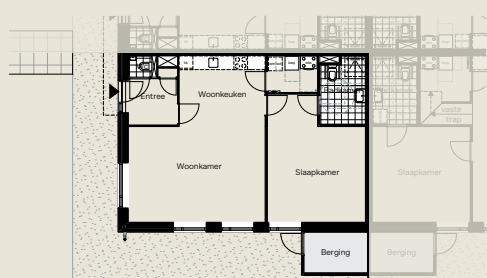
Begane grond
