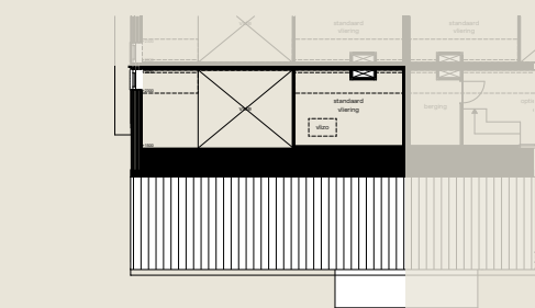
1e Verdieping
