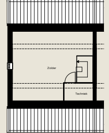
2e Verdieping
