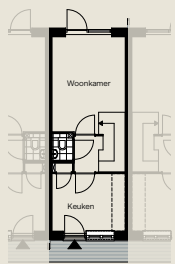
Begane grond
