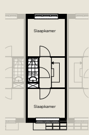
1e Verdieping
