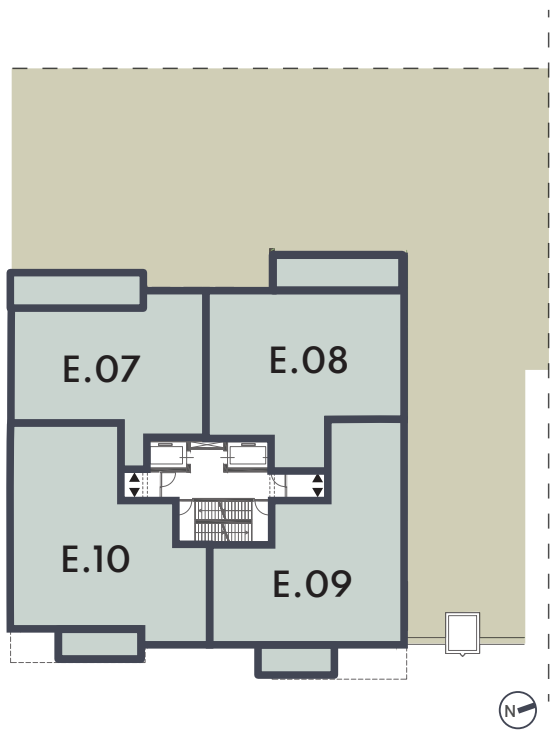
Vierde verdieping
