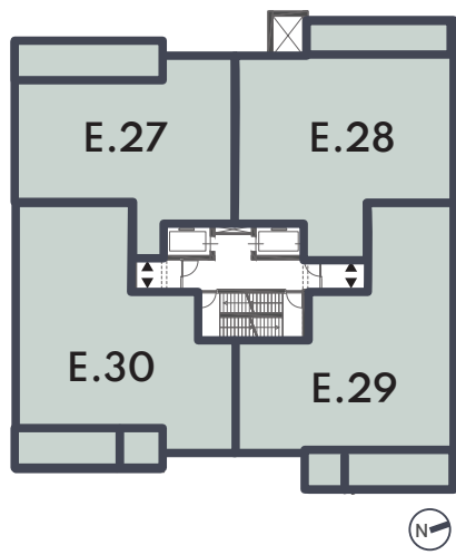
Negende verdieping
